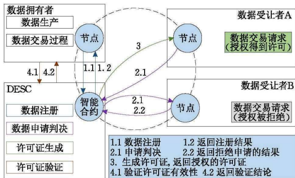
图 8 DESC [101] 工作流
