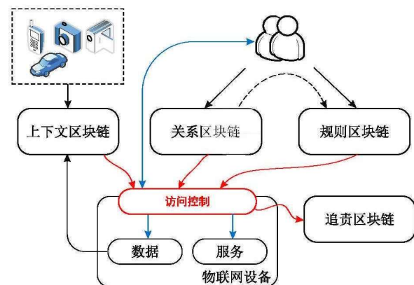
图 4 ControlChain [69] 架构
