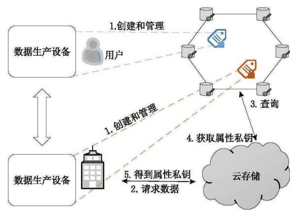
图 5 BaDS [76] 框架
