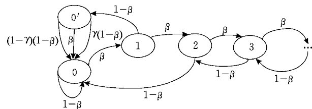
图 2 自私挖矿状态机
