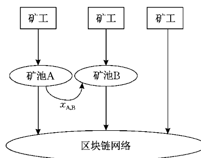
图 3 区块截留攻击场景
